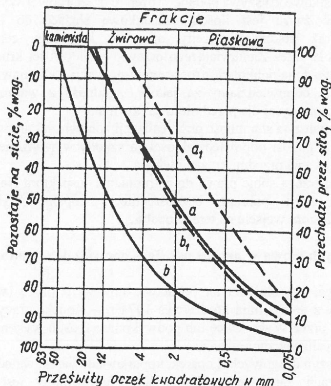
Tablica 1. Skład ramowy uziarnienia optymalnej mieszanki żwirowej
