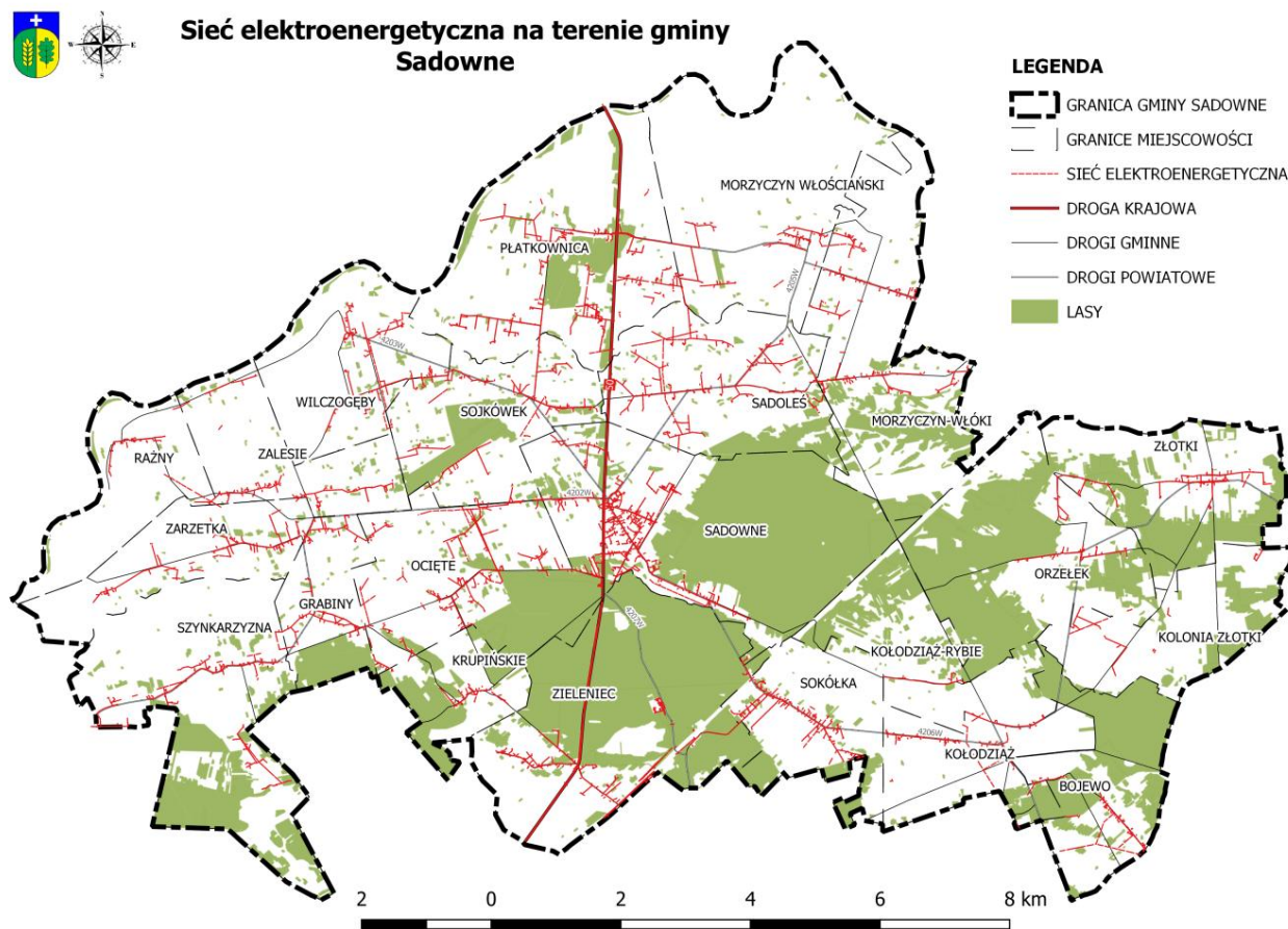
Ryc. 15.7 Sieć elektroenergetyczna na terenie gminy Sadowne
