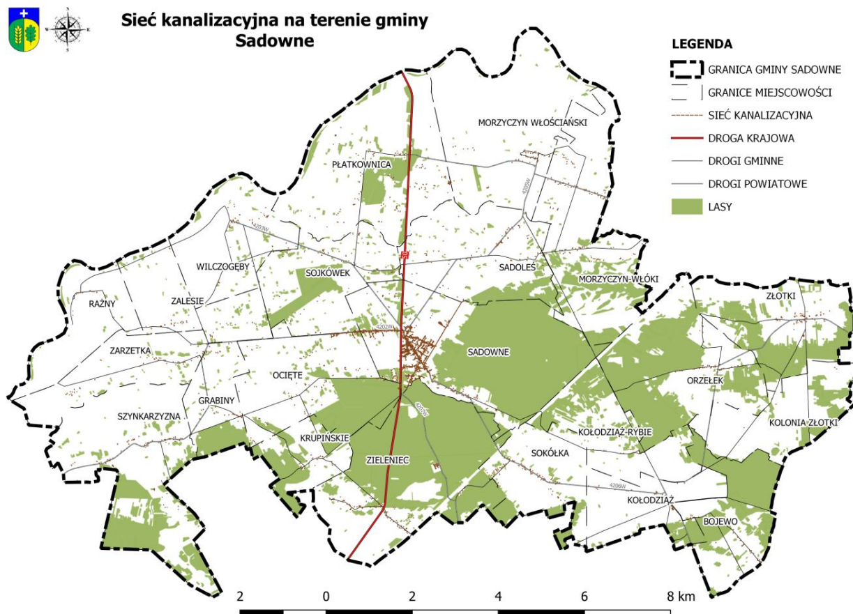
Ryc. 15.5 Sieć kanalizacyjna na terenie gminy Sadowne
